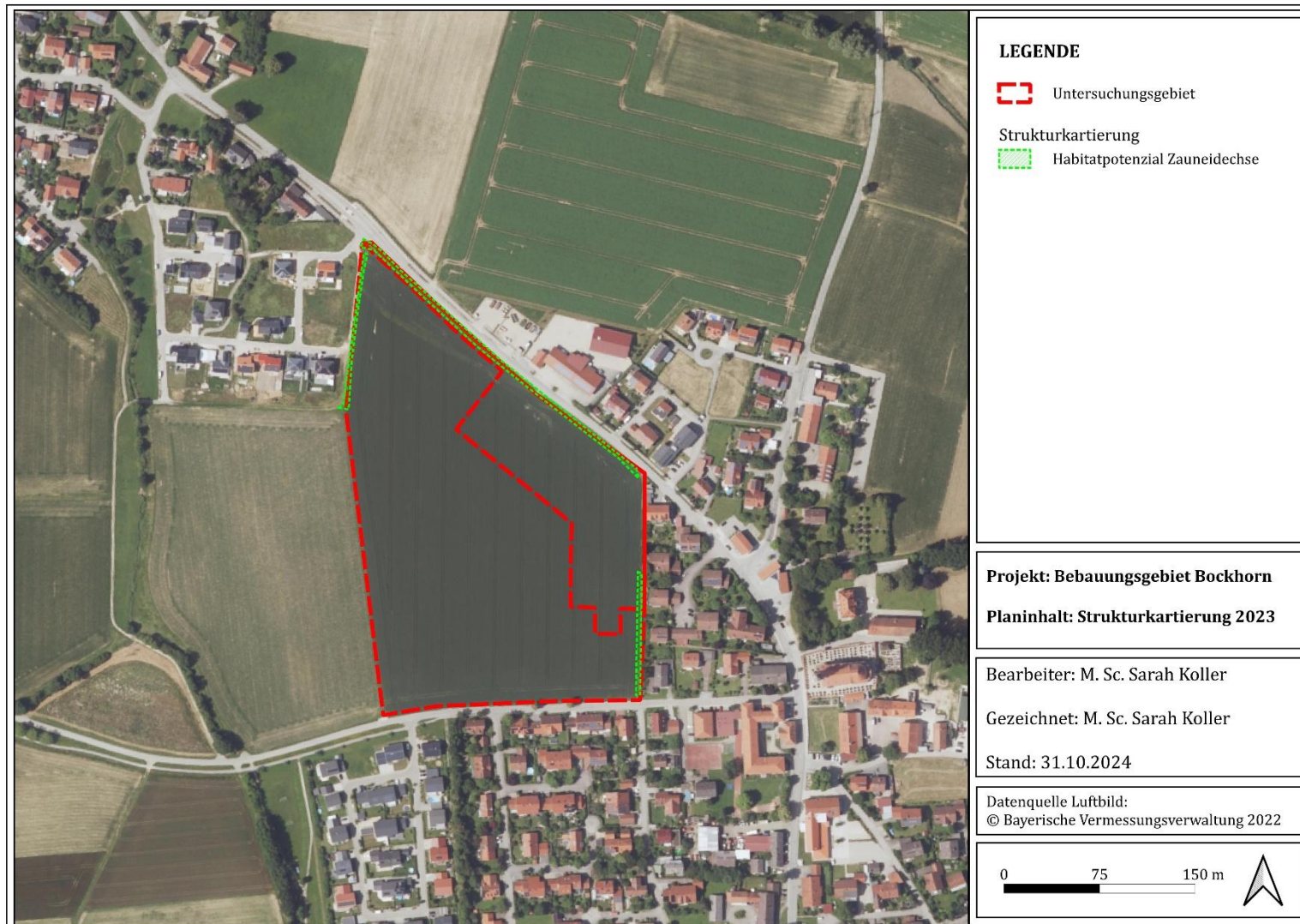
Abbildung 3: Strukturkartierung 2023.
